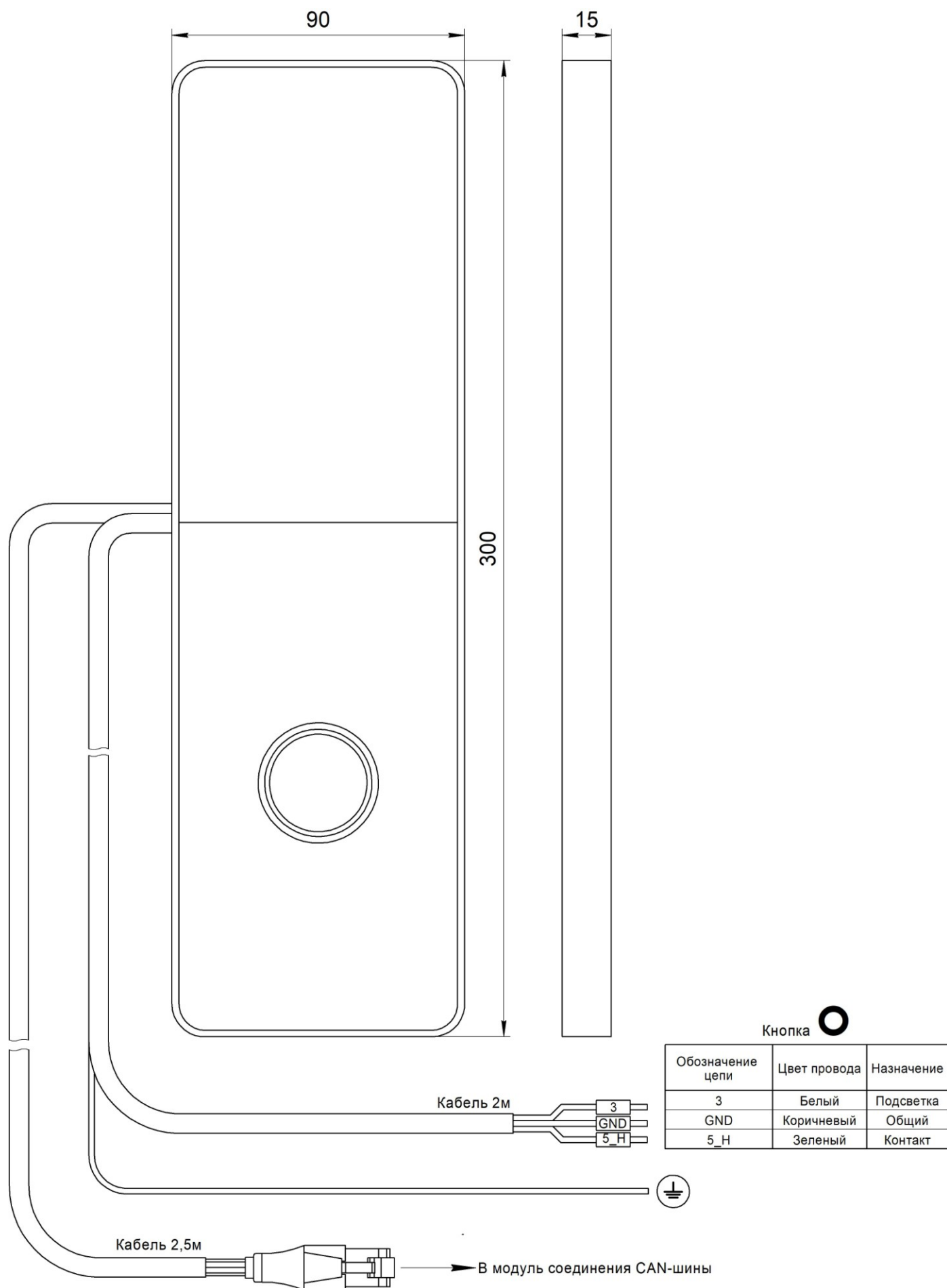
Рис.1 Внешний вид Вызывной пост ОНИКС (жгут RJ45) НШЕК.468381.014
